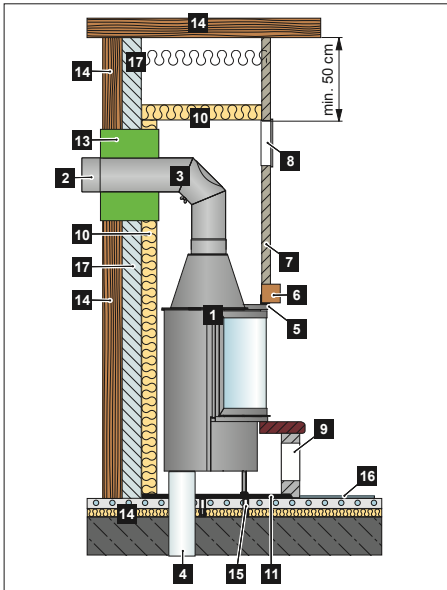
Ausführung bei brennbaren Anbauwänden
