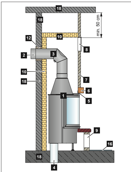
Ausführung bei nicht brennbaren Anbauwänden
